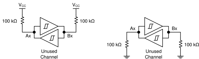
図 7-2. 未使用のトランシーバー チャネルの適切な終端
