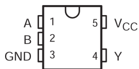
図 4-1. DCK パッケージ、5 ピン SOT-SC70 (上面図)
