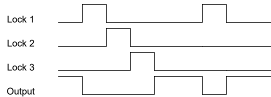
図 8-2. インターロック信号およびロジック出力
