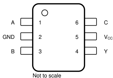
図 4-1. DCK パッケージ、6 ピン SC-70 (上面図)
