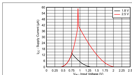
図 5-1. 入力電圧に対する電源電流、1.8V および 2.5V 電源
