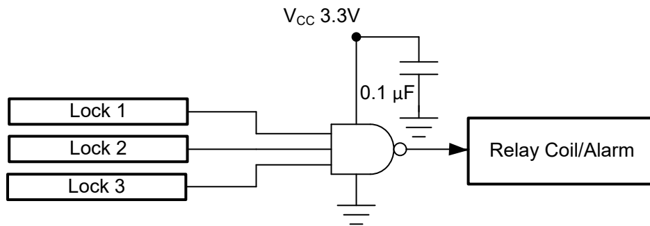
図 8-1. 代表的なアプリケーションの図
