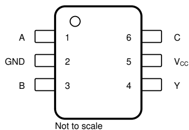
図 4-1. DCK または DBV パッケージ、6 ピン SC-70 または SOT-23 (上面図)
