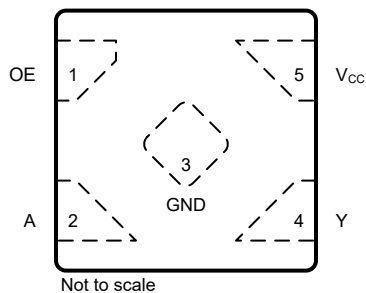
図 4-1. DTX パッケージ、 5 ピン X2SON (上面図)
