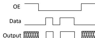
図 8-2. アプリケーション タイミング図
