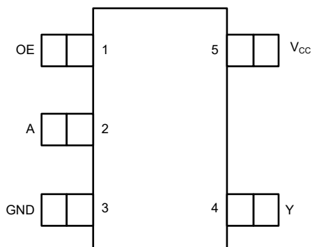
図 4-1. DCK パッケージ、 5 ピン SOT-SC70 (上面図)
