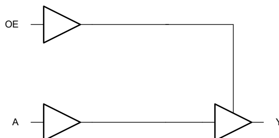
ロジック図
