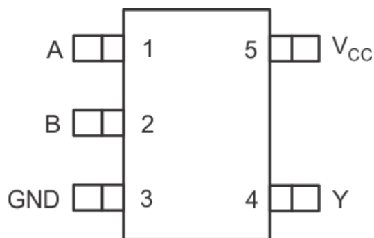
図 4-1. DCK、DBV パッケージ 5 ピン SC70、SOT-23 (上面図)
