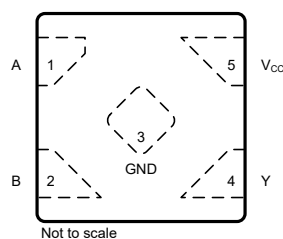
図 4-2. DTX パッケージ 5 ピン X2SON (上面図)
