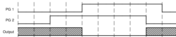
図 8-2. 代表的なアプリケーションのタイミング図
