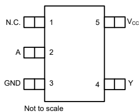
図 4-1. DCK、DBV パッケージ 5 ピン SC70、SOT-23 (上面図)
