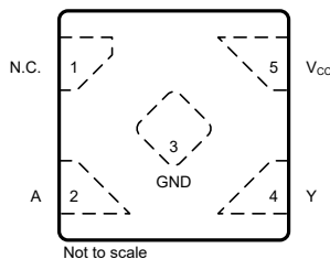
図 4-2. DTX パッケージ 5 ピン X2SON (上面図)
