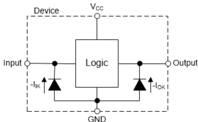
図 9-1. 各入力と出力に対するクランプ ダイオードの電気的配置
