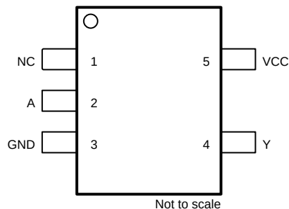
図 4-2. SN74LVC1G16-Q1 DCK パッケージ、5 ピン SOT-SC70 (上面図)
