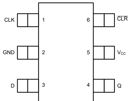
図 4-1. DBV または DCK パッケージ、6 ピン SOT-23 または SOT-SC70 (上面図)
