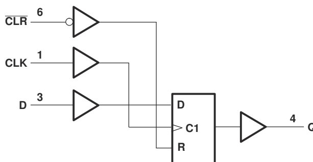
ロジック図
