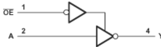
図 7-1. 論理図 (正論理)
