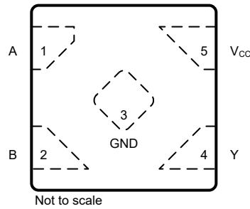
図 4-1. DTX パッケージ、 5 ピン X2SON (上面図)
