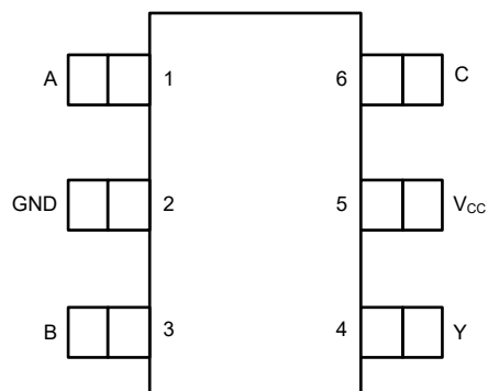
図 4-1. DBV または DCK パッケージ、6 ピン SOT-23 または SC-70 (上面図)
