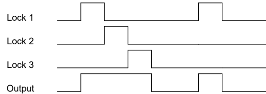
図 7-2. インターロック信号およびロジック出力
