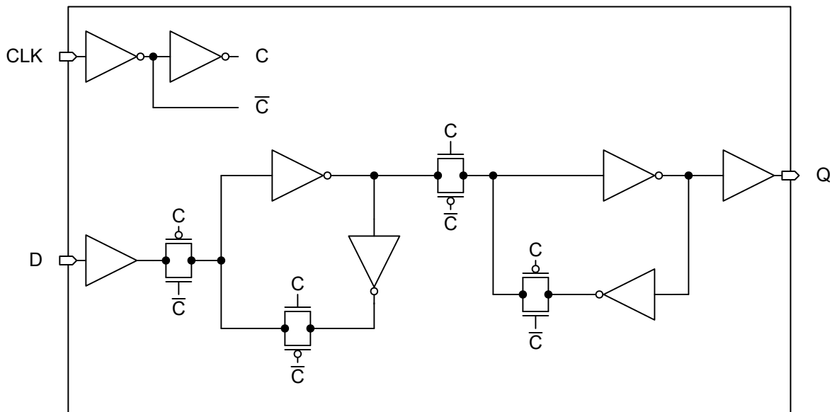
図 7-1. 論理図 (正論理)
