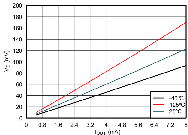
図 5-6. Low 状態における出力電圧と電流との関係、2.3V 電源
