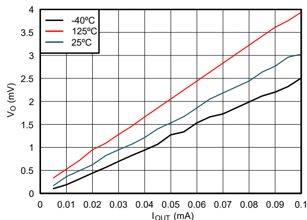
図 5-8. Low 状態における出力電圧と電流との関係、1.38V 電源
