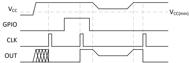
図 8-2. 電源電圧変更に伴うデータ保持
