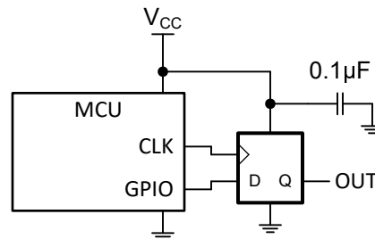
図 8-1. 代表的なアプリケーション回路図
