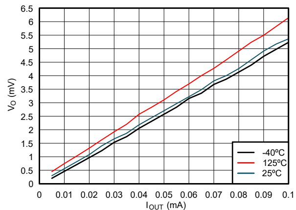
図 5-9. Low 状態における出力電圧と電流との関係、1.1V 電源
