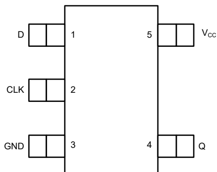
図 4-1. DBV パッケージ、 5 ピン SOT-23 (上面図)
