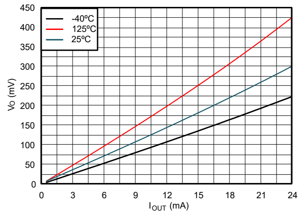
図 5-5. Low 状態における出力電圧と電流との関係、3V 電源
