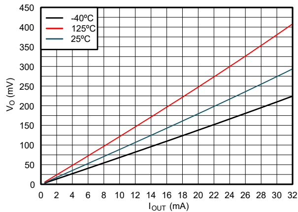
図 5-4. Low 状態における出力電圧と電流との関係、4.5V 電源
