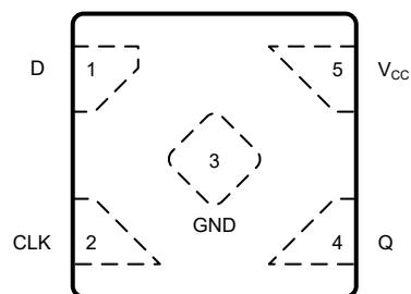
図 4-2. DTX パッケージ、 5 ピン X2SON (透過上面図)
