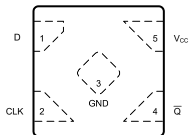
図 4-2. DTX パッケージ、 5 ピン X2SON (上面図)
