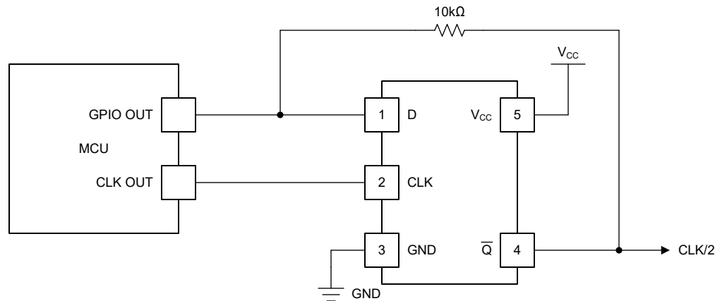
図 8-1. 代表的なアプリケーション回路図
