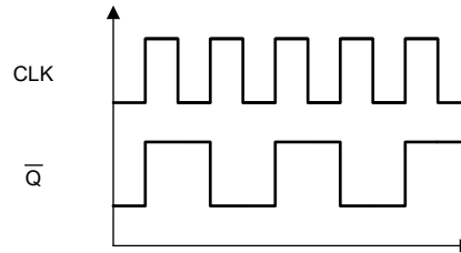
図 8-2. 代表的なアプリケーションのタイミング図
