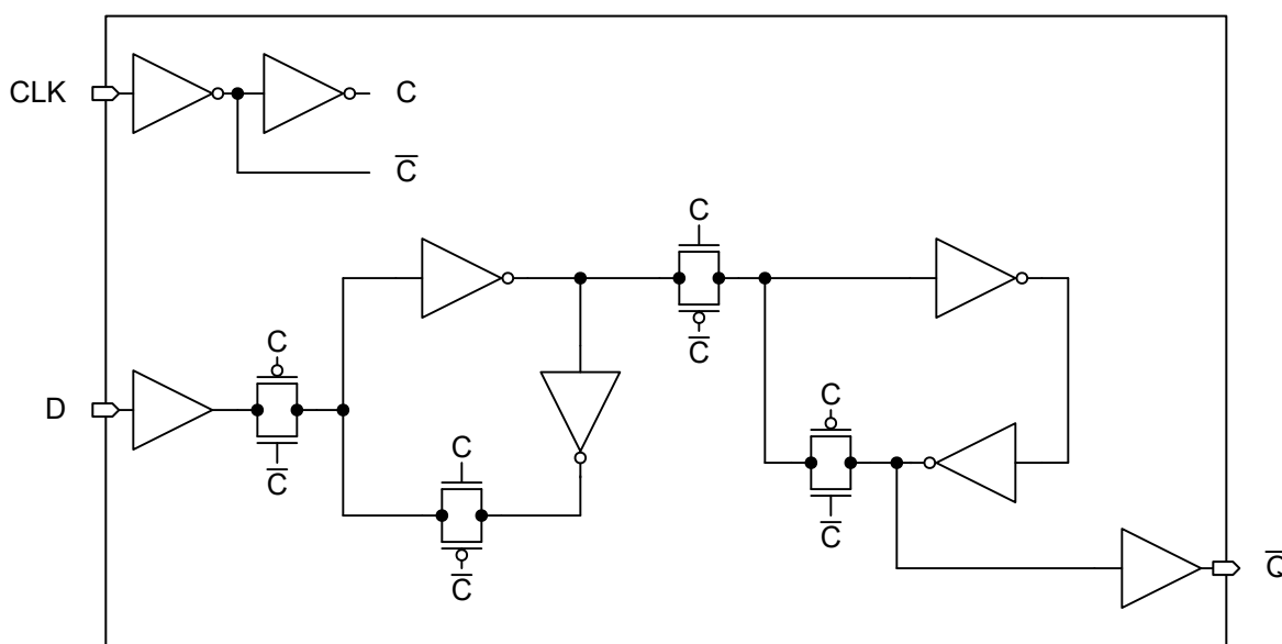
ロジック図
