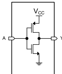
図 7-1. 機能図
