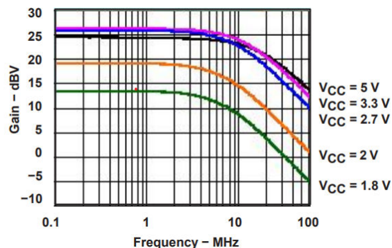
図 8-3. オープンループ ゲイン特性
