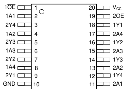
図 4-2. SN74LVC240A-Q1 PW、DGS パッケージ（上面図）
