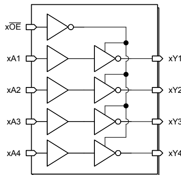
図 7-1. SN74LVC240A-Q1 の論理図 (正論理)
