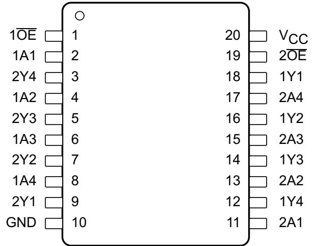
図 4-2. DB、DGV、DW、N、NS、DGS および PW パッケージ 20 ピン SSOP、TVSOP、SOIC、PDIP、SO、VSSOP および TSSOP 正面図
