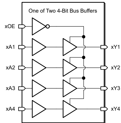
論理図 (正論理)
