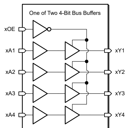
論理図 (正論理)
