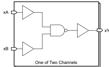
論理図 (正論理)
