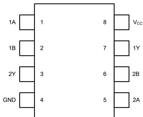
図 4-1. DCT パッケージ 8 ピン SSOP 上面図
