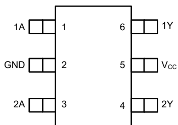
図 4-1. DCK、DBV パッケージ 5 ピン SC70、SOT-23 (上面図)
