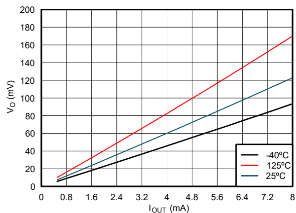
図 5-5. Low 状態における出力電圧と電流との関係、2.3V 電源
