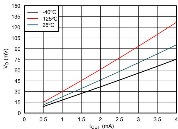
図 5-6. Low 状態における出力電圧と電流との関係、1.65V 電源
