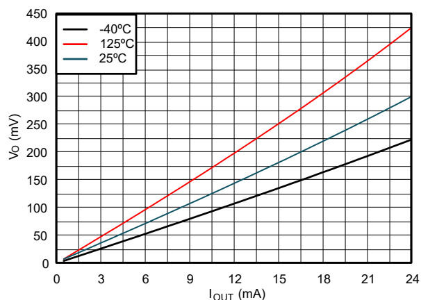
図 5-4. Low 状態における出力電圧と電流との関係、3V 電源
