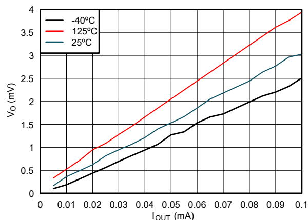
図 5-7. Low 状態における出力電圧と電流との関係、1.38V 電源
