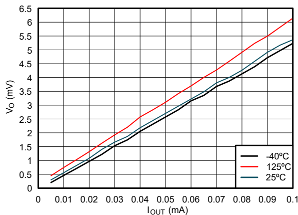
図 5-8. Low 状態における出力電圧と電流との関係、1.1V 電源
