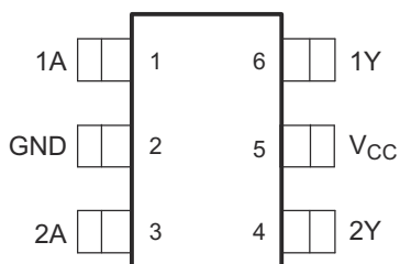
図 3-1. DBV または DCK パッケージ、6 ピン SOT-23 または SC70 (上面図)
