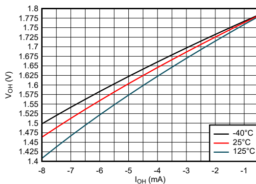
図 5-7. High 状態における出力電圧と電流との関係、1.8V 電源
