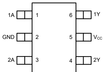
図 4-1. DBV、6 ピン SOT-23 (上面図)
