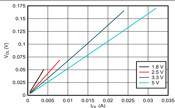
図 5-3. Low 状態における出力電圧と電流との関係
