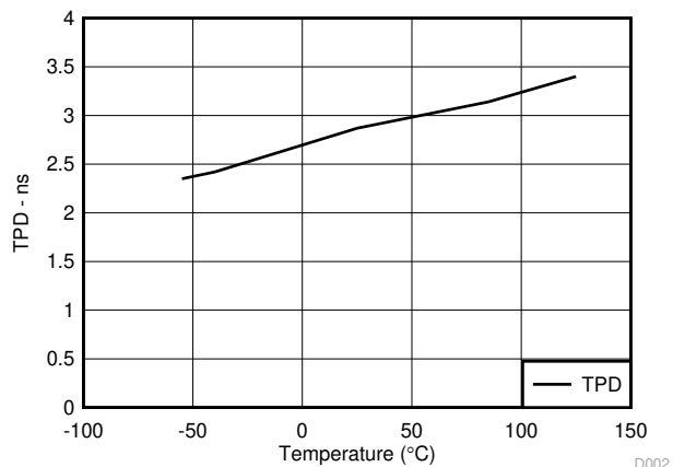
図 5-2. 3.3V での温度範囲における SN74LVC541A TPD
