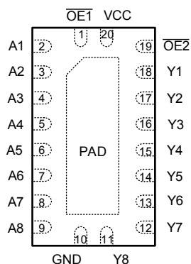
図 4-3. SN74LVC541A RKS パッケージ (上面図)
