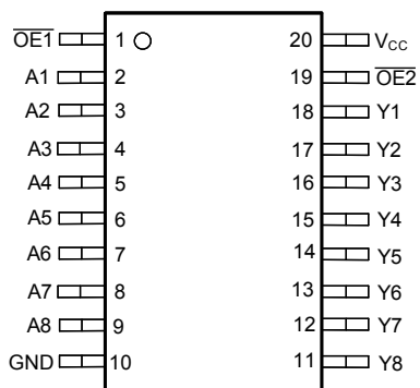
図 4-1. SN54LVC541A J または W パッケージ (上面図)
