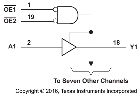
図 7-1. 論理図 (正論理)
