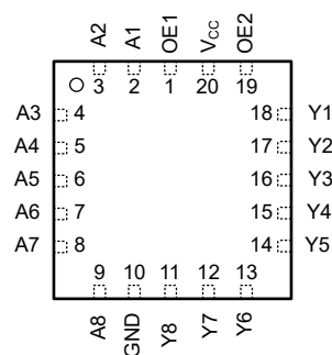
図 4-2. SN54LVC541A FK パッケージ (上面図)
