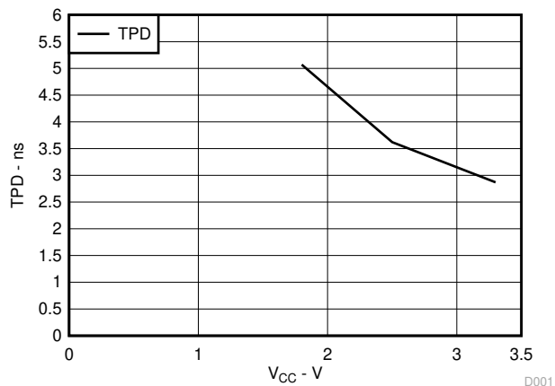
図 5-1. 25°Cでの V_{CC} における SN74LVC541A TPD
