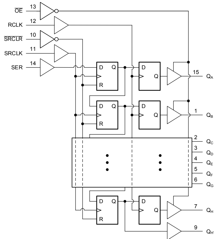
図 7-1. SN74LVC595A-Q1 の論理図 (正論理)
