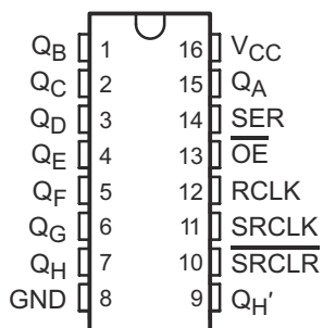
図 4-1. PW パッケージ 16 ピン TSSOP (上面図)
