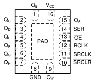
図 4-2. BQB パッケージ、16 ピン WQFN (上面図)
