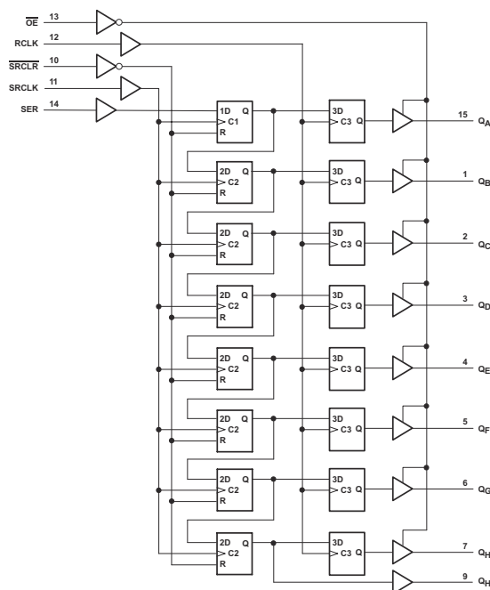
論理図 (正論理)
