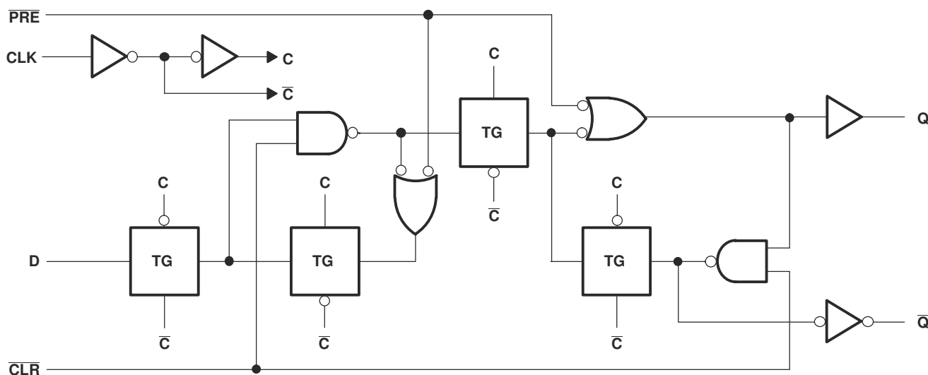
図 6-1. 論理図、各フリップフロップ (正論理)
