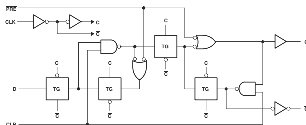
論理図、各フリップフロップ (正論理)
