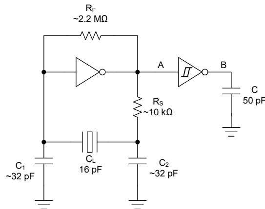
図 8-1. 代表的なアプリケーション回路図
