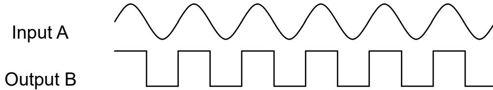
図 8-2. シュミット トリガ正弦波入力および方形波出力
