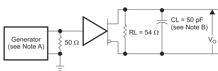
図 6-2. ドライバ V_{OD3}
