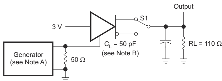
図 6-3. ドライバテスト回路と電圧波形
