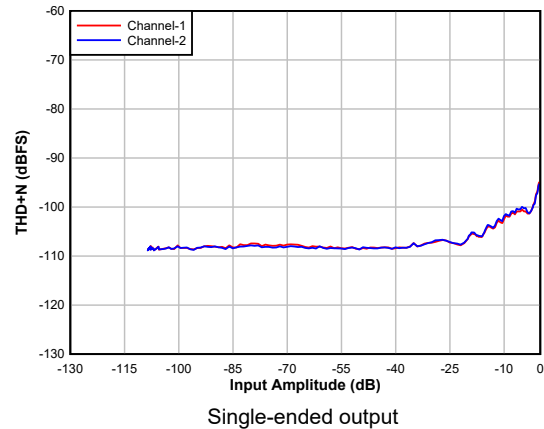
図 5-6. DAC THD+N Level vs Input
