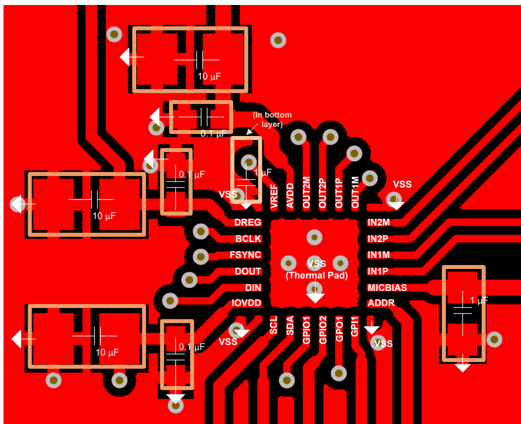
図 8-5. Example Layout
