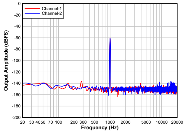
图 8-2. DAC FFT with -60dBFS Input
