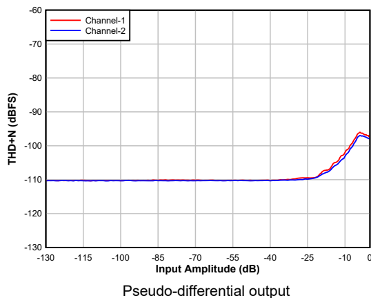
図 5-7. DAC THD+N Level vs Input
