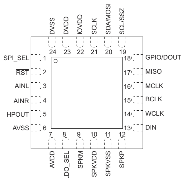
図 4-1. RGE Package 24-Pin VQFN Top View
