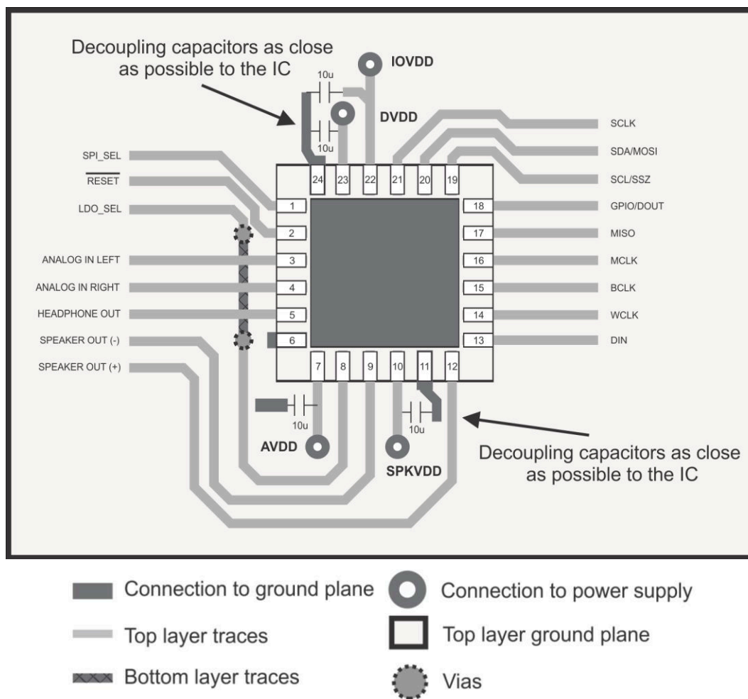
図 9-5. Layout Diagram
