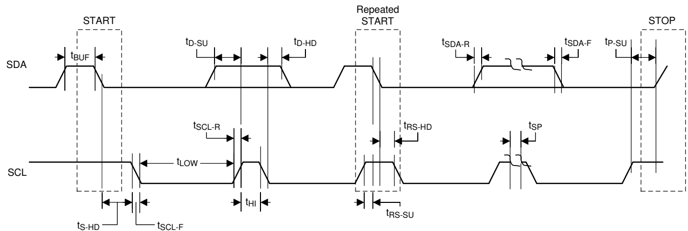
図 6-4. I²C 通信ポート タイミング図
