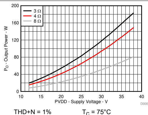
図 6-8. 出力電力と電源電圧との関係
