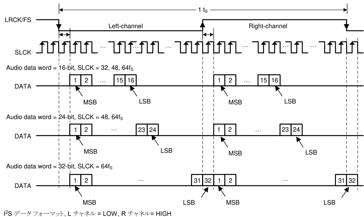
図 7-5. I 2 S オーディオ データ形式
