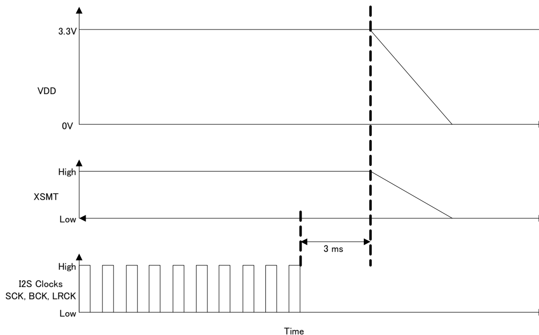
図 7-16. シリアル ポート ミューティングのタイミング図
