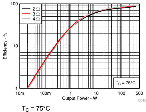
図 6-17. 効率と出力電力との関係
