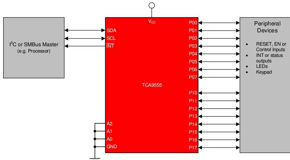
概略回路図
