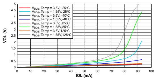
図 5-1. V_{DD2} レベル = 3.6V、1.65V、 T_A = -40^\circ C 、 25^\circ C 、 85^\circ C 、 125^\circ C での SDA 出力低電圧 ( V_{OL} ) と負荷電流 ( I_{OL} ) との関係
