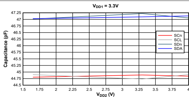
図 5-3. 25^\circ C における、ターゲットチャネル (SCn/SDn) 容量 ( C_{IO (OFF)} ) と電源電圧 ( V_{DD2} ) との関係
