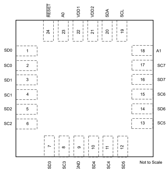
図 4-2. RGE パッケージ、24 ピン VQFN (上面図)
