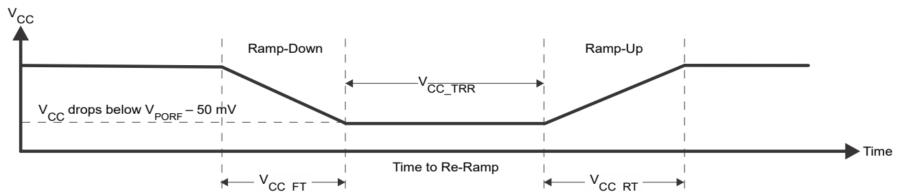
図 8-4. パワーオン リセットの波形
