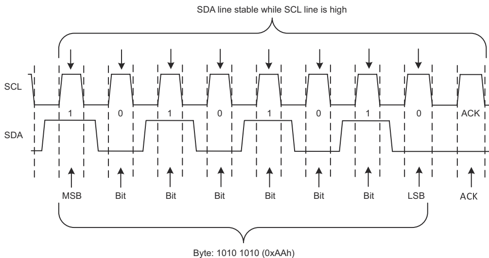
図 7-2. ビット転送
