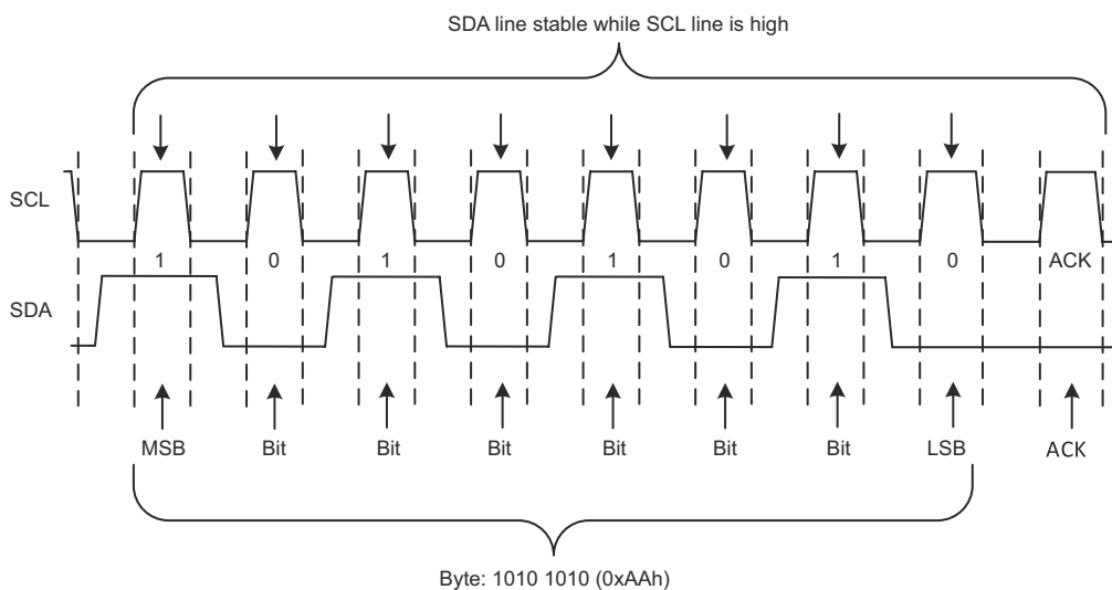
図 7-2. ビット転送
