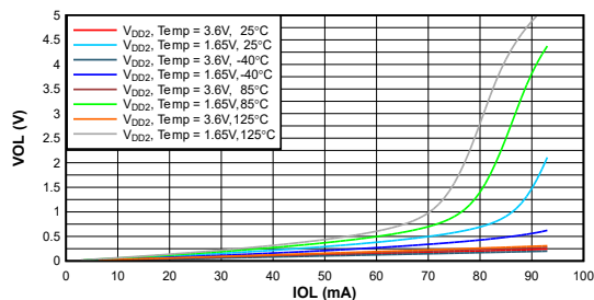
図 5-1. V_{DD2} レベル = 3.6V、1.65V、 T_A = -40^\circ C 、 25^\circ C 、 85^\circ C 、 125^\circ C での SDA 出力低電圧 ( V_{OL} ) と負荷電流 ( I_{OL} ) との関係
