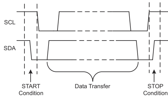
図 7-1. START 条件と STOP 条件の定義
