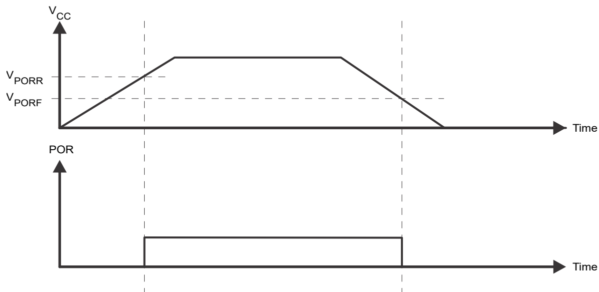
図 8-6. V_{POR}
