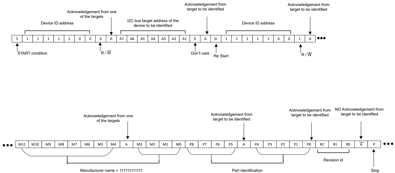
図 7-6. デバイス ID
