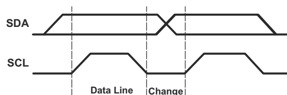
図 7-5. ビット転送
