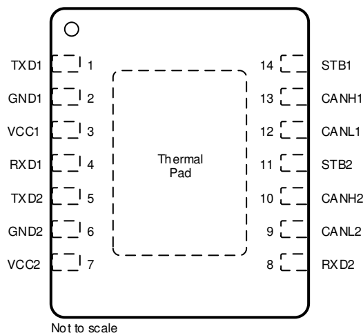
FIG 5-2. DMT Package TCAN1046-Q1, 14 Pin VSON, Top View
