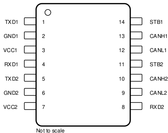
FIG 5-1. D Package TCAN1046-Q1, 14 Pin SOIC, Top View
