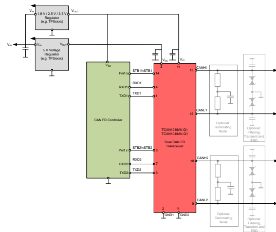
概略回路図
