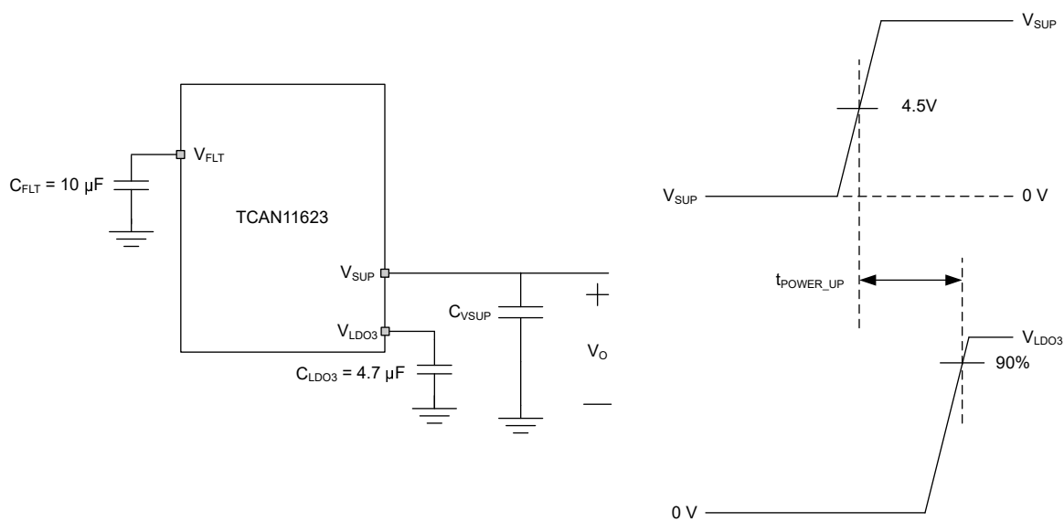
図 6-9. TCAN11623 t_{POWER\_UP} 時間測定
