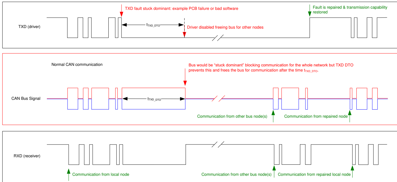
図 7-4. TXD DTO のタイミング図
