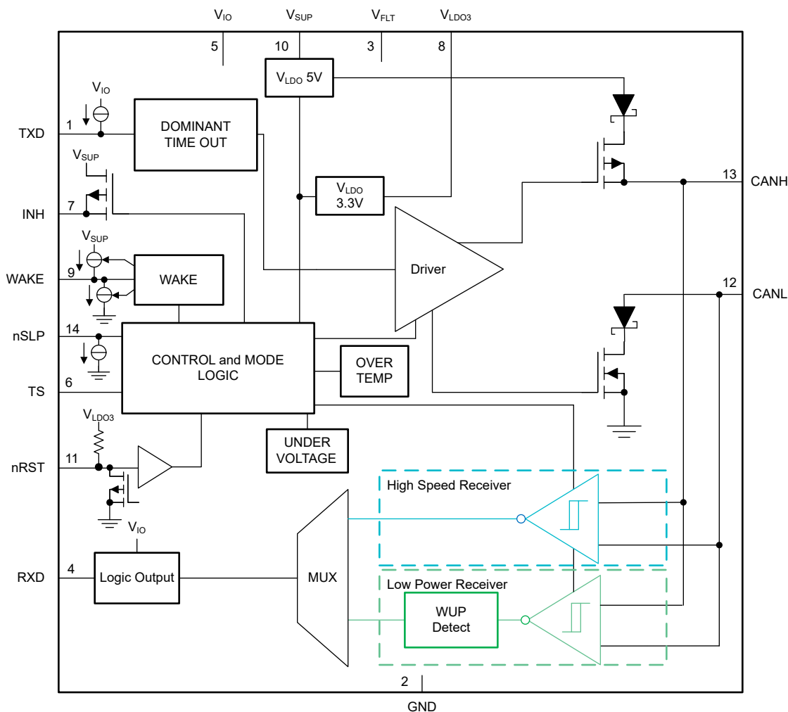
图 7-2. TCAN11623-Q1
