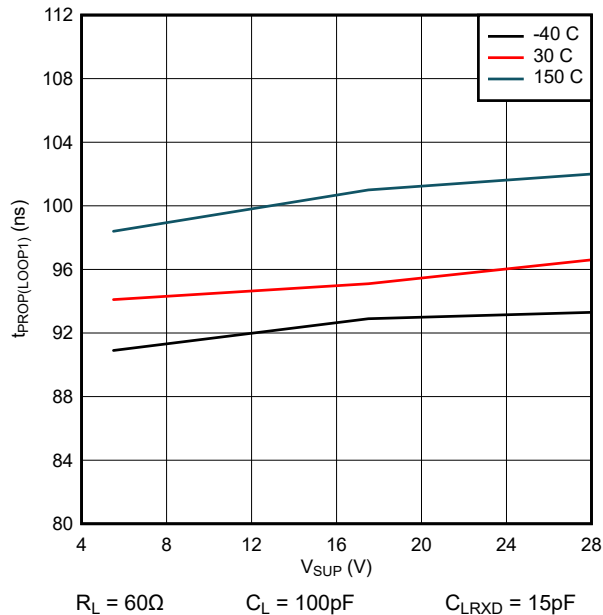
図 5-1. V SUP 上の t PROP(LOOP1)
