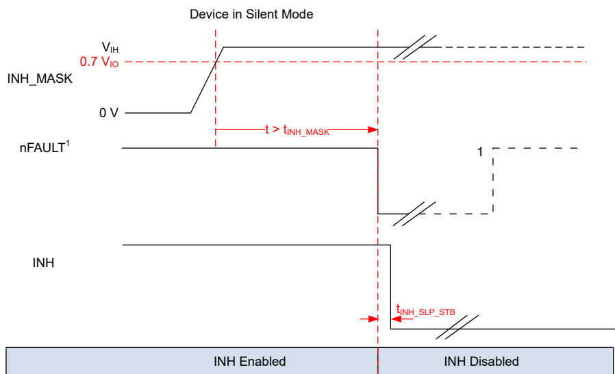
図 6-10. INH ディセーブルのタイミング図
