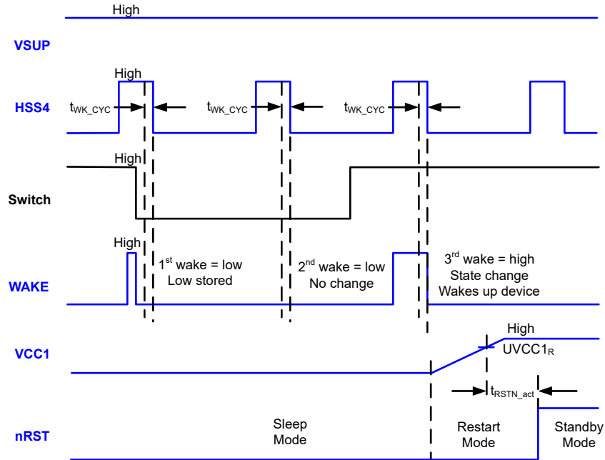
図 8-23. サイクリックセンシングのタイミング図
