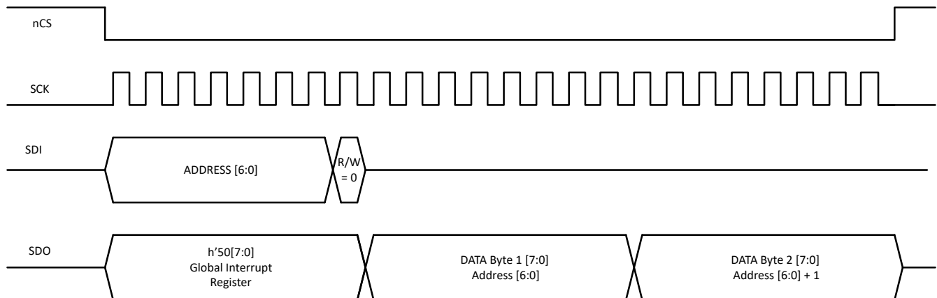
図 8-10. SPI 読み出し (2 バイトモード)
