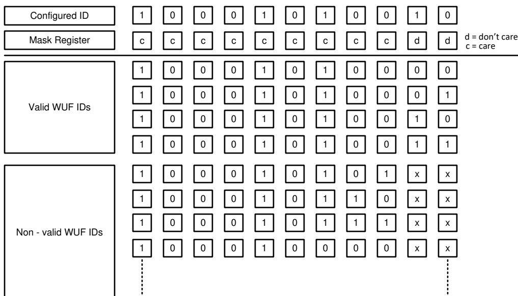
図 8-24. WUF の ID と ID マスクの例
