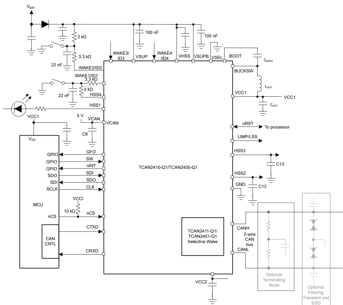
図 8-22. サイクリックセンシング構成のアプリケーション図
