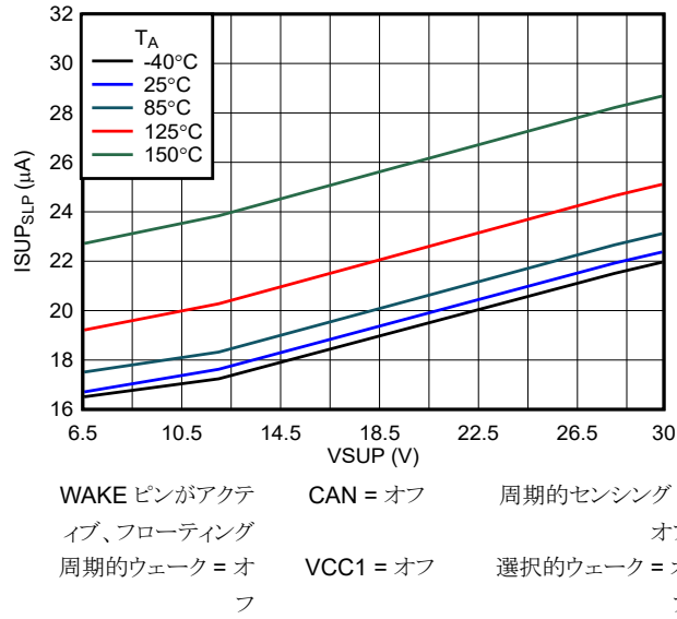
図 6-1. スリープ モードのバッテリー消費電流と VSUP および温度との関係
