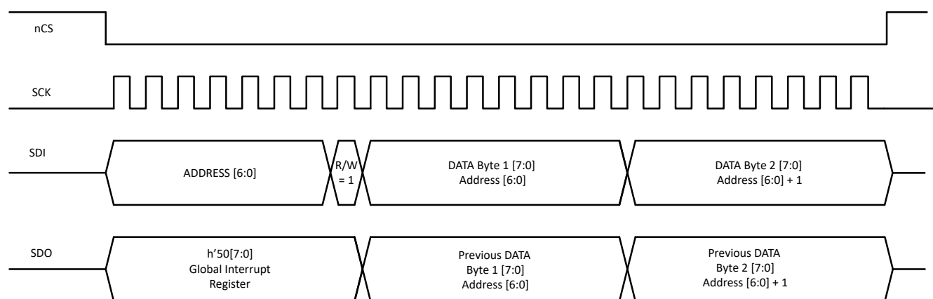
図 8-11. SPI 書き込み (2 バイトモード)
