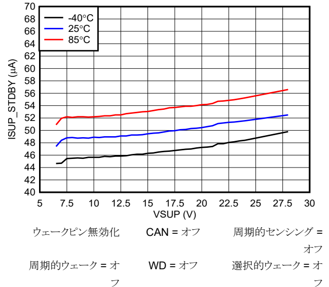
図 6-2. スタンバイ モードのバッテリー消費電流と VSUP および温度との関係
