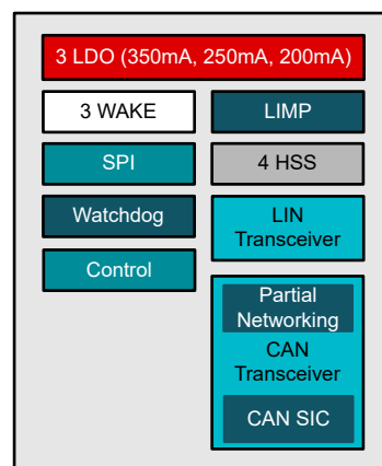
TCAN2847-Q1 の図
