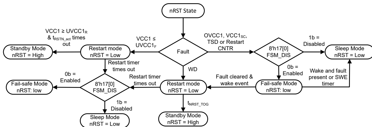
図 8-5. nRST 状態図
