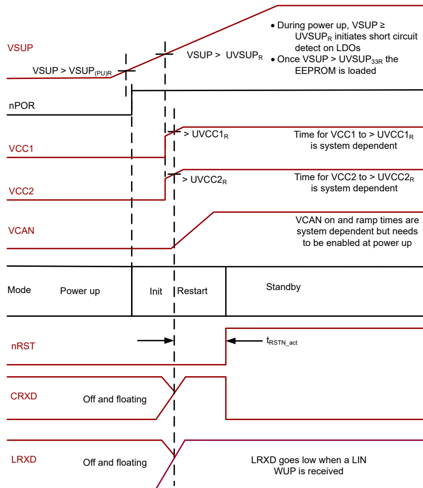
図 7-18. 起動タイミング
