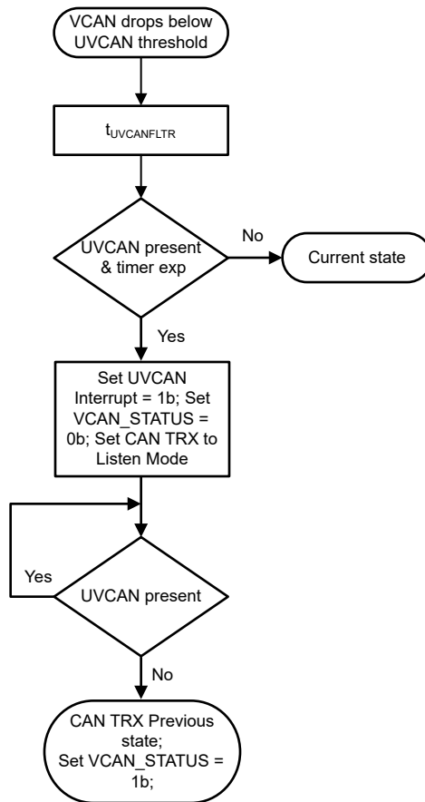
図 8-50. UVCAN 状態図
