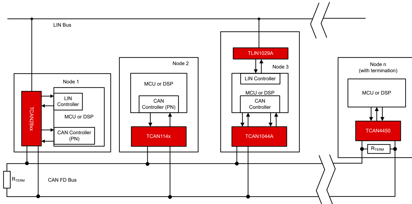
概略回路図
