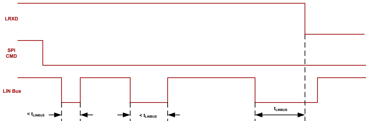
図 8-45. バス フォルトなし：バスリセッсп条件とウェイクアップによるスリープモードへの移行
