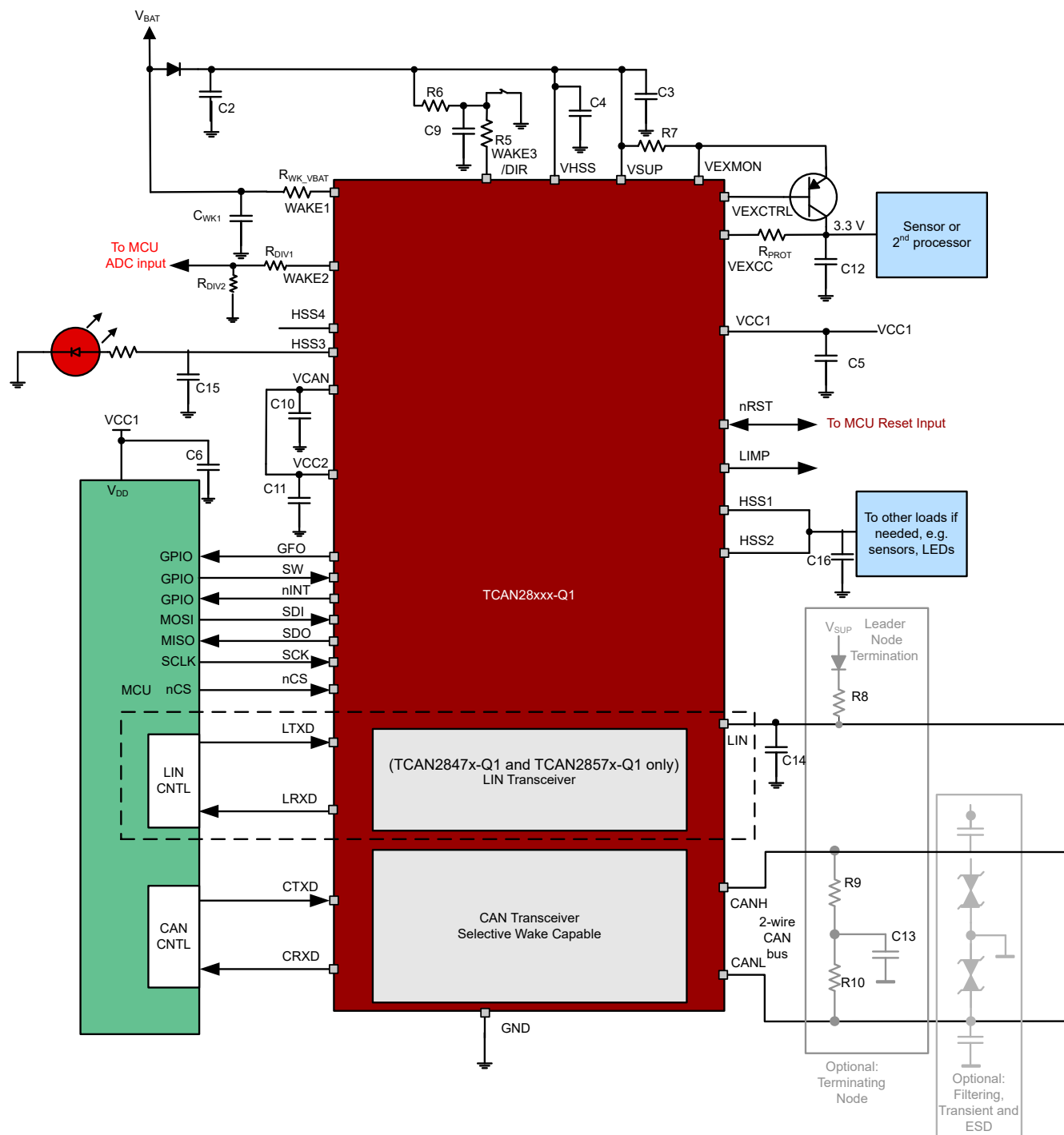
図 10-13. WAKE1 ピンと WAKE2 ピン間で VBAT 監視機能をイネーブにした代表的なアプリケーション図
