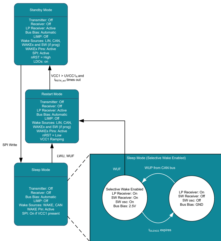
図 8-20. 選択的ウェーク有効時のスリープモード
