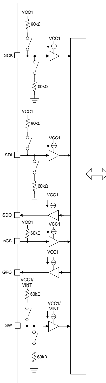
図 8-2. デジタル入力および出力のブロック図
