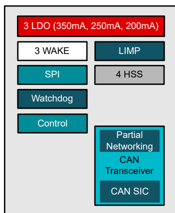
TCAN2845-Q1 の図
