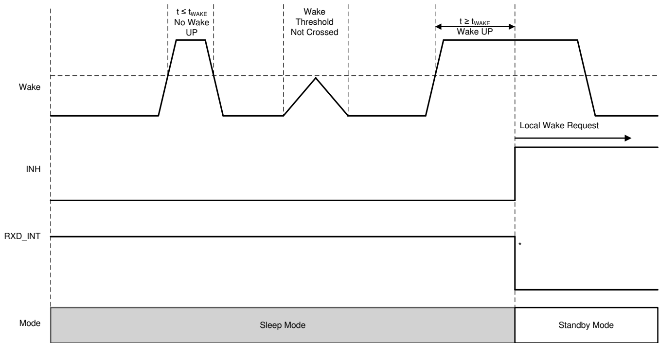
図 26. Local Wake Up – Rising Edge
