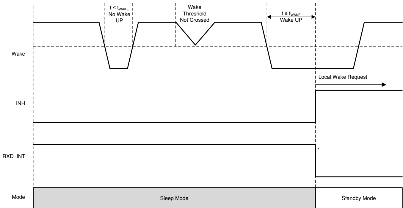
図 27. Local Wake Up – Falling Edge
