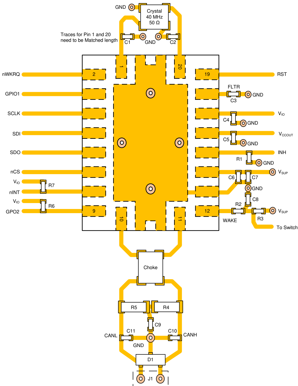
✎ 113. Example Layout
