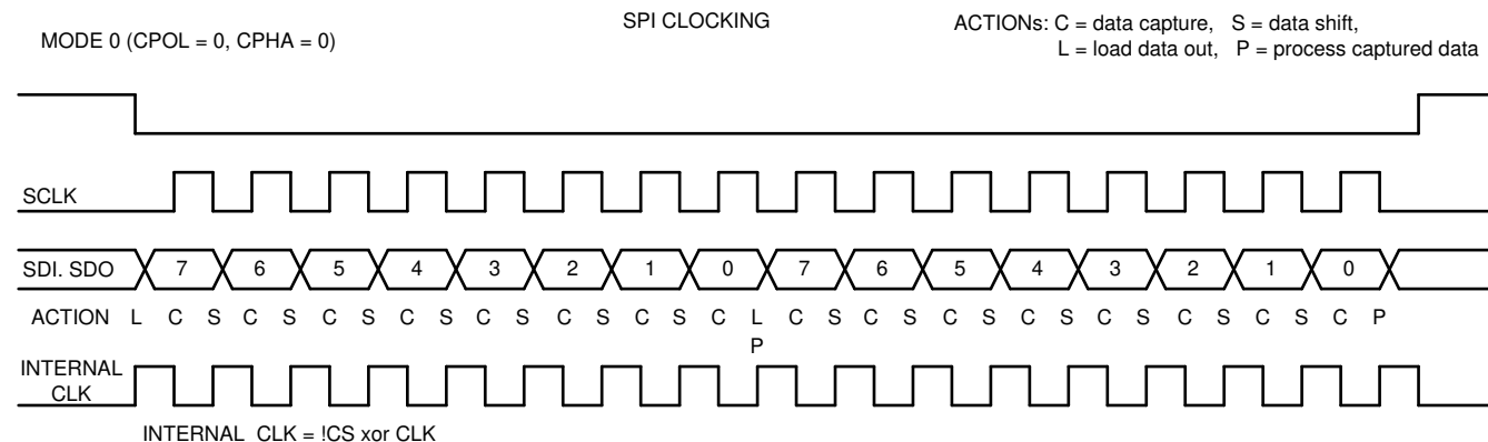
図 34. SPI Clocking
