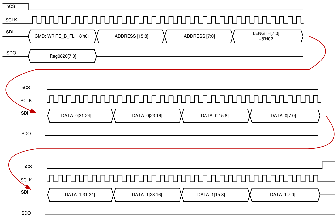
图 35. Write
