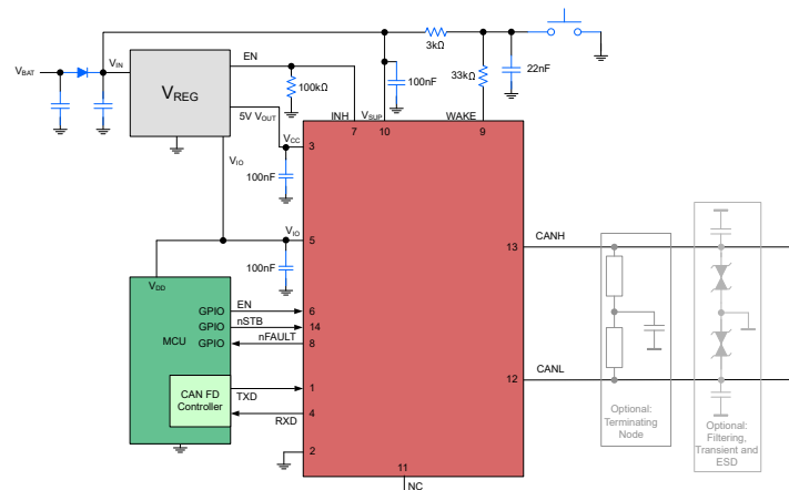
概略回路図
