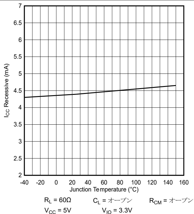
図 5-2. I_{CC} リセッシブと温度との関係
