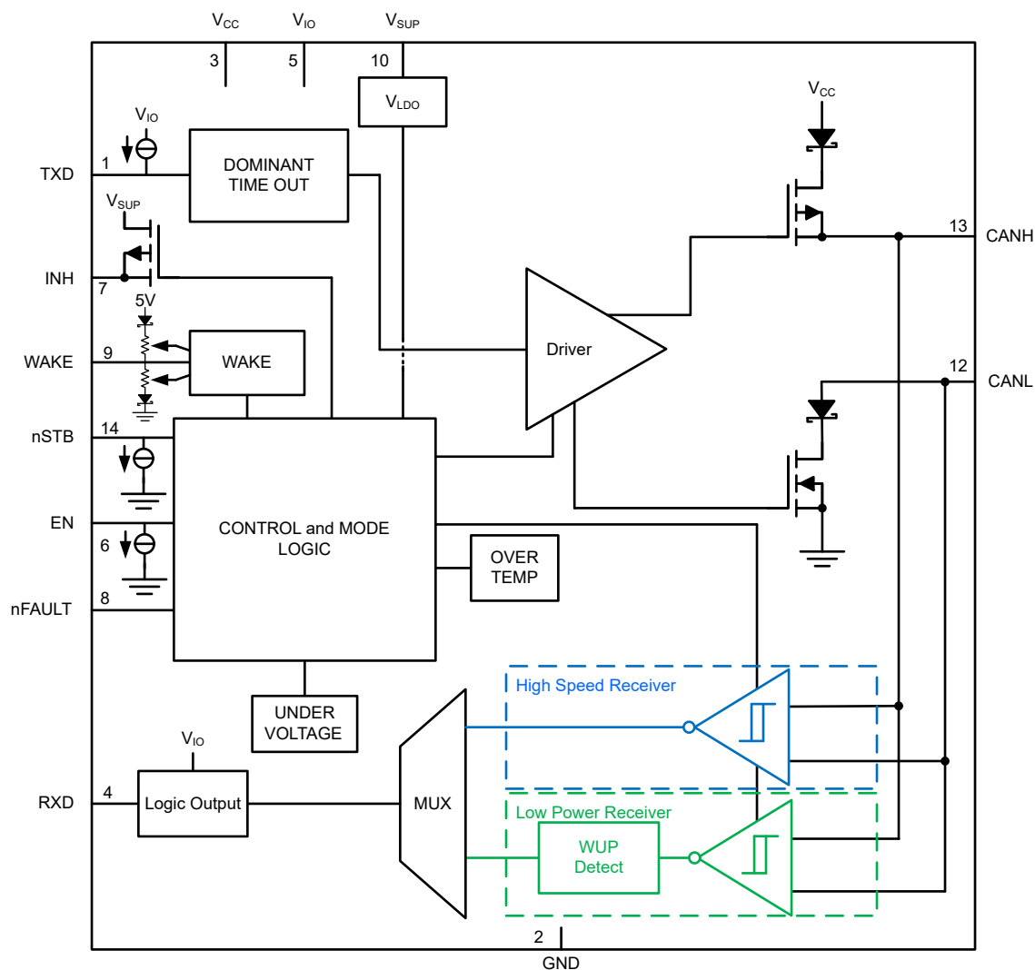
図 7-1. TCAN943-Q1 機能ブロック図
