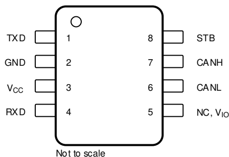
図 5-1. DDF パッケージ、8 ピン SOT (上面図)
