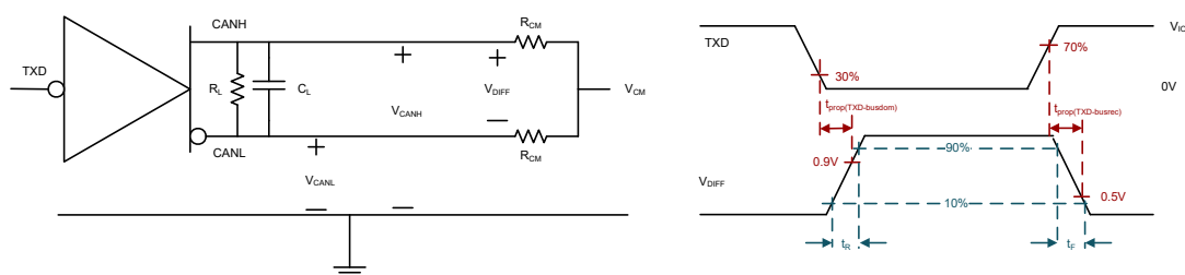
図 7-2. ドライバテスト回路と測定
