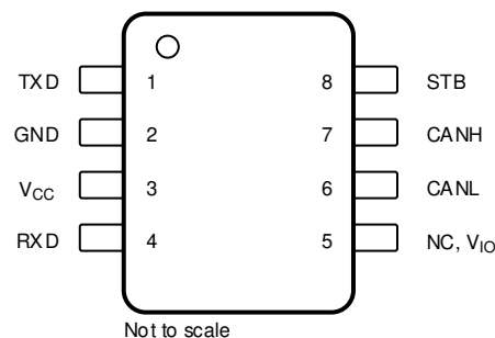
図 5-2. D パッケージ、8 ピン SOIC (上面図)
