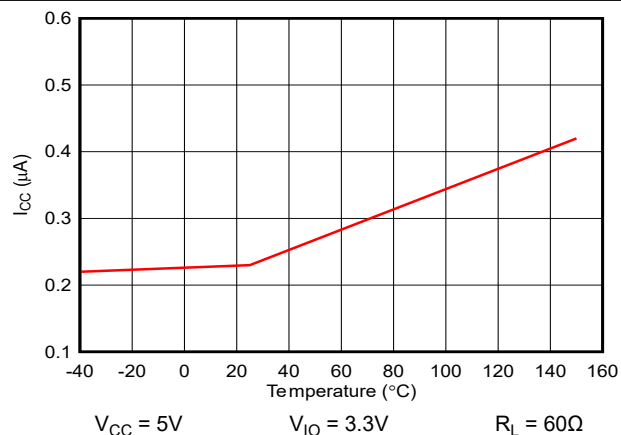
図 6-2. I_{CC} サイレントと温度との関係
