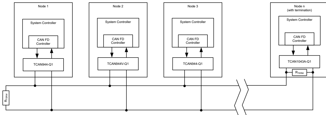
図 9-3. 代表的な CAN バス
