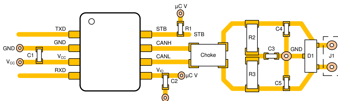
図 9-6. レイアウト例
