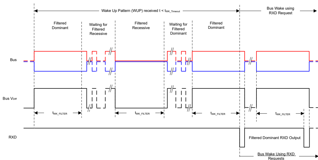
図 8-4. t_{WK\_TIMEOUT} によるウェークアップパターン (WUP)
