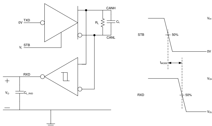
図 7-5. t_{MODE} テスト回路と測定
