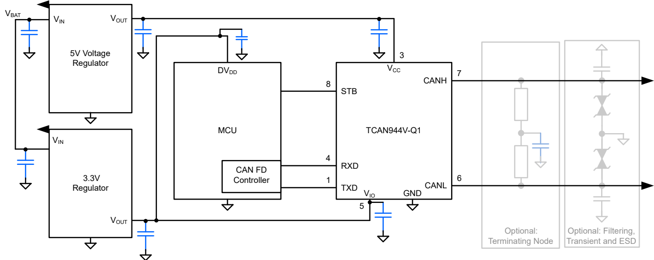
図 9-5. 3.3V の IO 接続を使用した標準的なトランシーバアプリケーション
