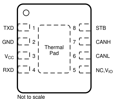
図 5-3. DRB パッケージ、8 ピン VSON (上面図)
