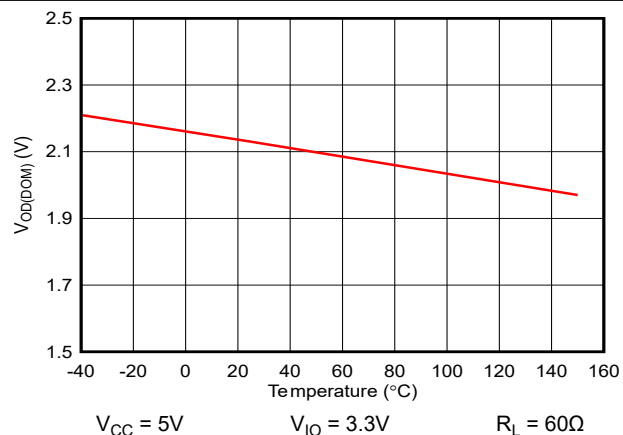
図 6-1. V_{OD(DOM)} と温度との関係
