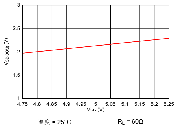
図 9-4. V_{OD(DOM)} と V_{CC} との関係
