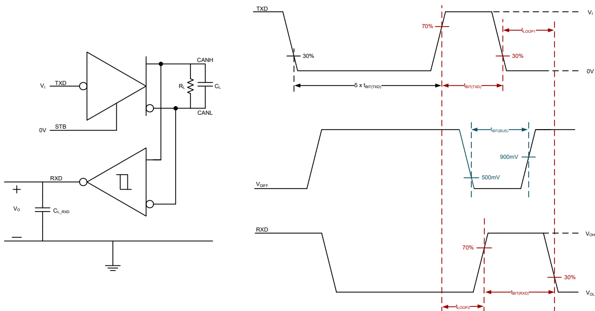
図 7-4. トランスミッタとレシーバのタイミング テスト回路と測定
