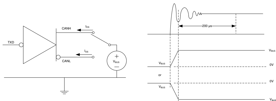
図 7-7. ドライバ短絡電流テスト回路と測定
