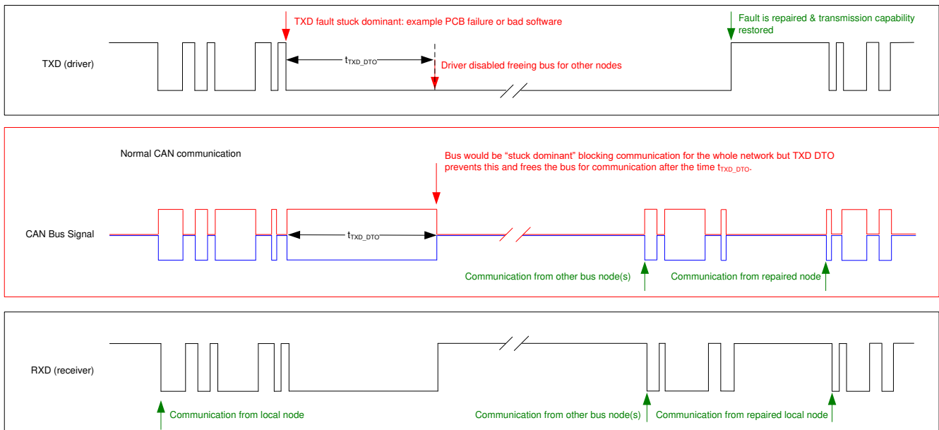
図 8-3. TXD ドミナントタイムアウトのタイミング図の例
