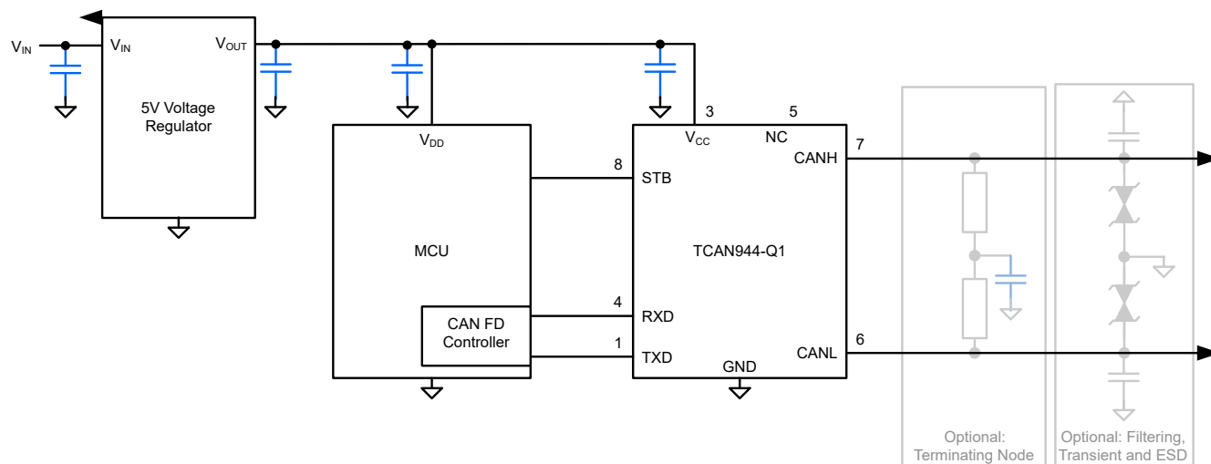
図 9-1. 5V の IO 接続を使用したトランシーバ アプリケーション
