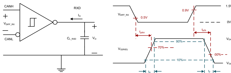
図 7-3. レシーバのテスト回路と測定
