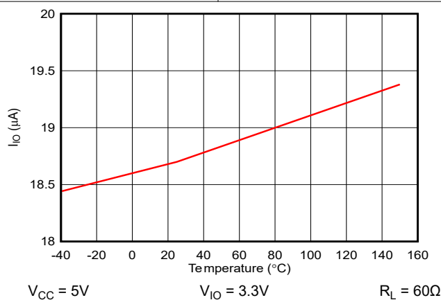
図 6-3. I_{IO} サイレントと温度との関係
