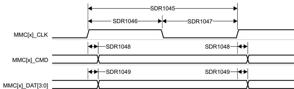
図 6-99. MMC1 – UHS-I SDR104 – 送信モード
