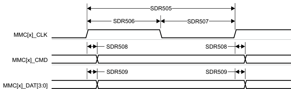
図 6-97. MMC1 – UHS-I SDR50 – 送信モード
