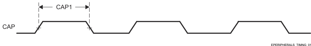
図 6-46. eCAP の入力タイミング
