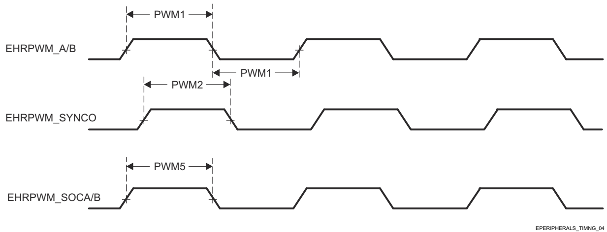
図 6-49. EPWM_A/B_out、ePWM_SYNCO、および ePWM_SOC A/B 入力タイミング
