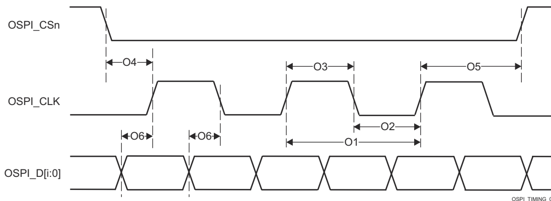
図 6-104. OSPI0/I のスイッチング特性 - PHY DDR データ トレーニング
