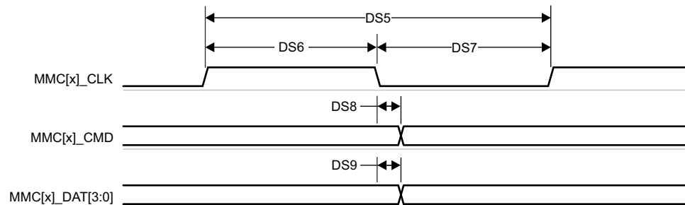
図 6-90. MMC1 – デフォルト速度 – 送信モード
