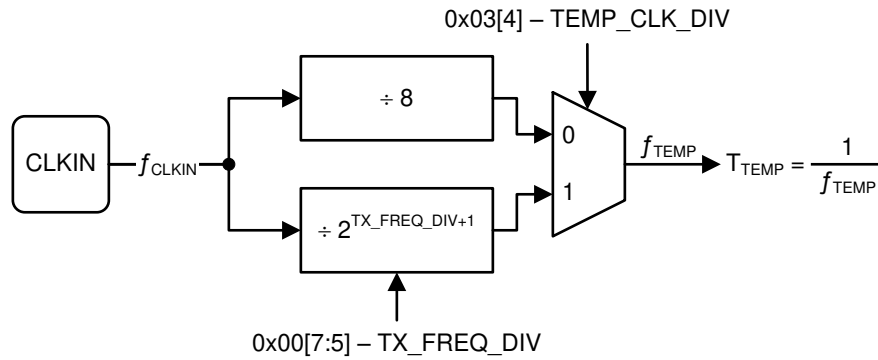
図 8-10. 温度測定のコック・ソース
