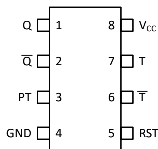
ピン配置図
